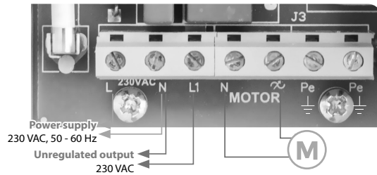
Fig. 1 Wiring diagrams
